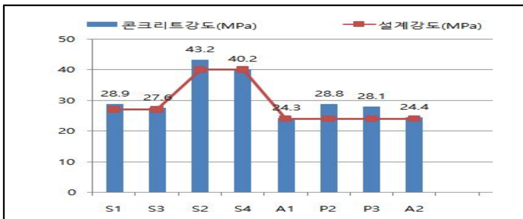
【그림 4.3】 압축강도 자료 비교·분석
