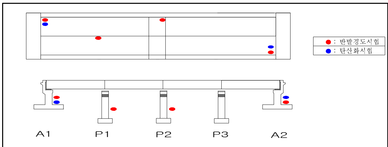
【그림 4.1】 내구성조사 및 시험 위치도
