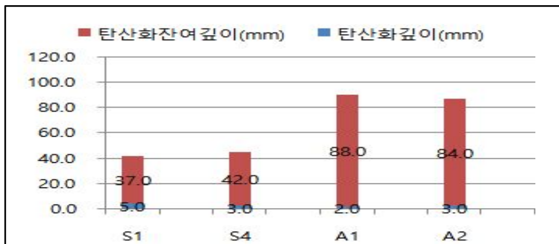
【그림 4.4】 탄산화 진행깊이 및 잔여깊이 측정결과
